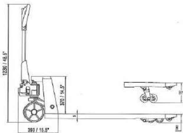
AC PERFIL SUPERBAJO 35
